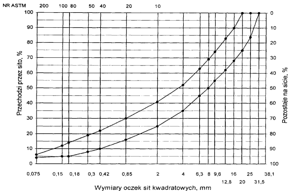
Rzędne krzywych granicznych uziarnienia MM w zależności od kategorii ruchu
