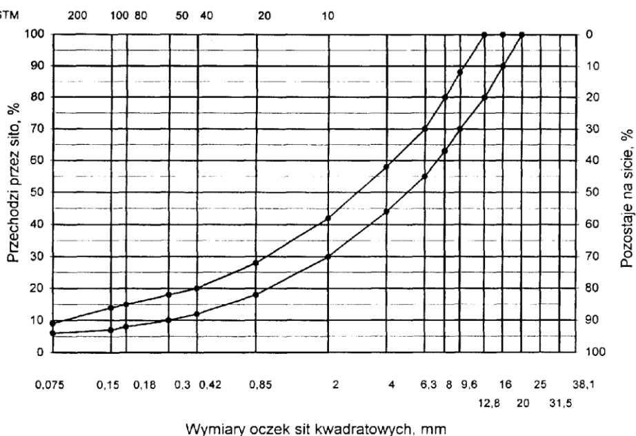
Rys. 3. Krzywe graniczne uziarnienia mieszanki mineralnej BA od 0 do 16 mm do warstwy ścieralnej nawierzchni drogi o obciążeniu ruchem KR4
