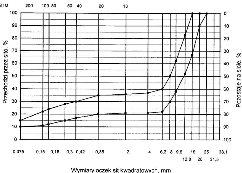
Rys. 2. Krzywe graniczne uziarnienia mieszanki mineralnej BA od 0 do 20 mm (mieszanka o nieciągłym uziarnieniu) do warstwy ścieralnej nawierzchni drogi o obciążeniu ruchem KR4
