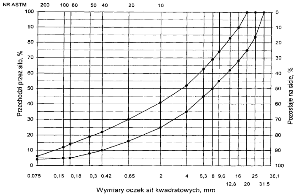
Rys. 6. Krzywe graniczne uziarnienia mieszanki mineralnej BA od 0 do 20 mm do warstwy wiążącej, wyrównawczej i wzmacniającej nawierzchni drogi o obciążeniu ruchem KR4
