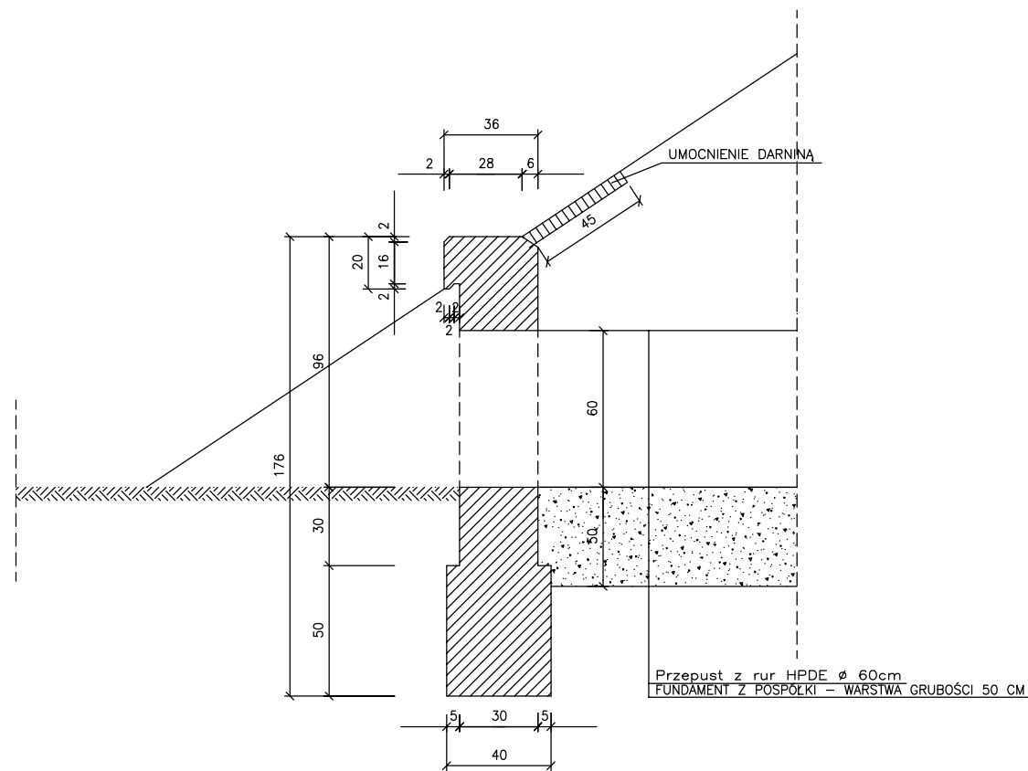
SZCZEGÓŁ ŚCIANKI CZOŁOWEJ
